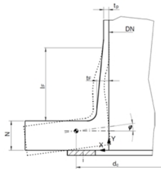
Figuur 26.7: Deformatie van flensaansluitingen
