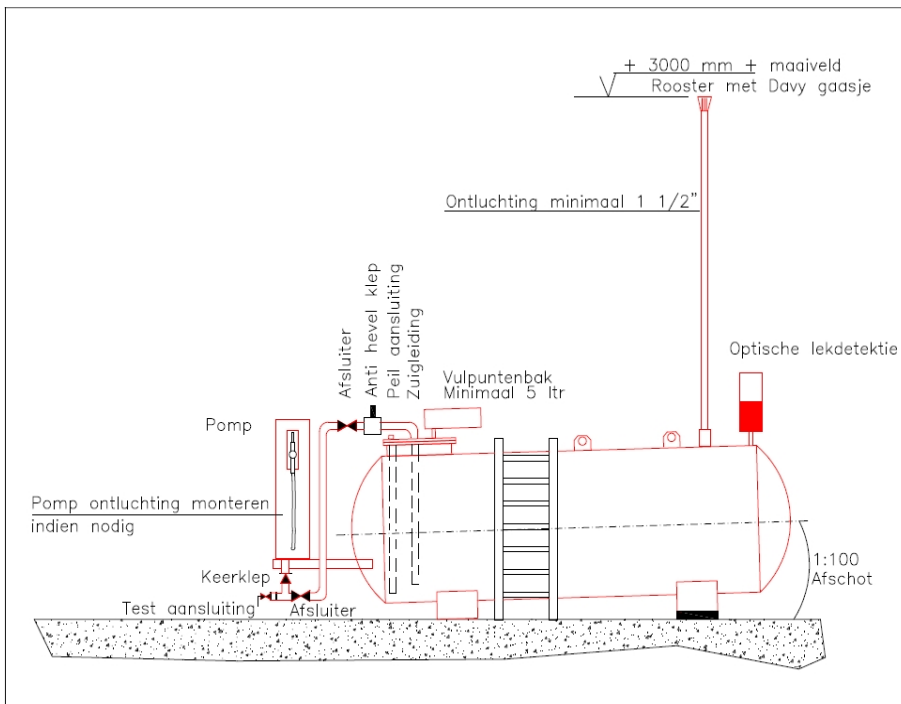
Figuur 13.1: Voorbeeld van antihevelvoorziening in bovengrondse tankinstallatie
