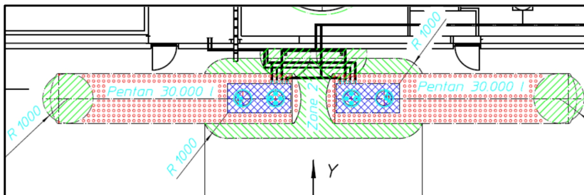
Figuur VI.6 – Voorbeeld van Ondergrondse pentaantanks (bovenaanzicht)
