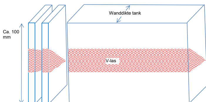
Figuur 26.2 Deel van de testplaat (100 x 100 mm met extrusielas)
