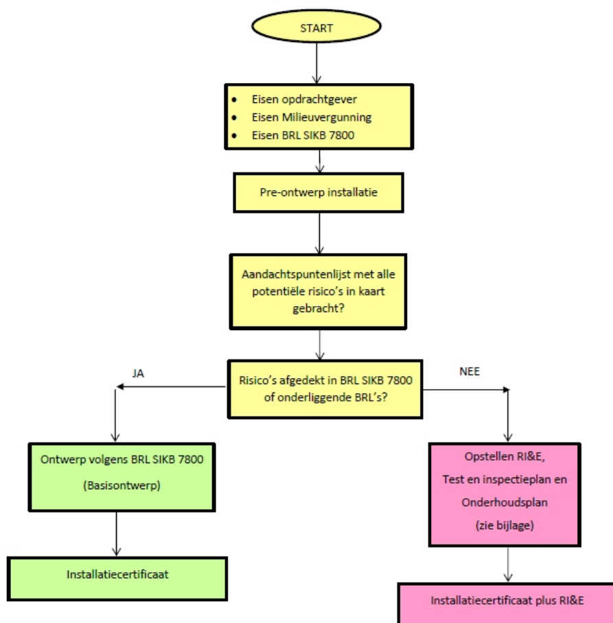
Figuur 7.1: Het ontwerp van een tankinstallatie
