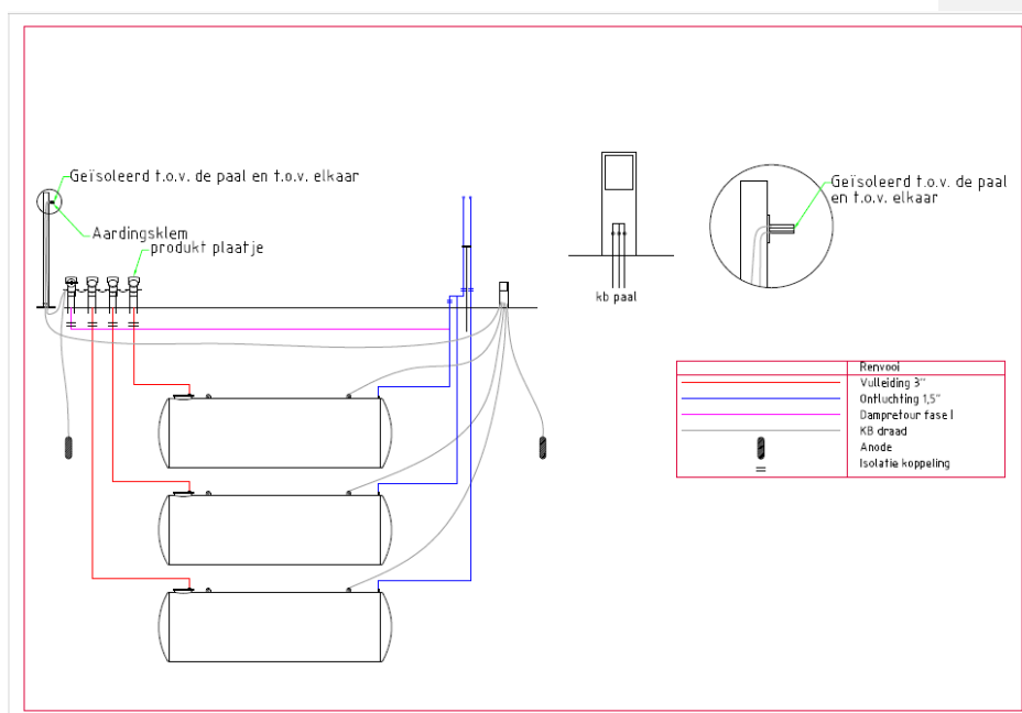
Figuur 16.1: Overzicht potentiaalvereffening/aarding bij tankinstallatie
