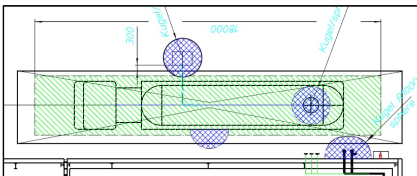
Figuur VI.7 – Voorbeeld van Tankauto (bovenaanzicht)
